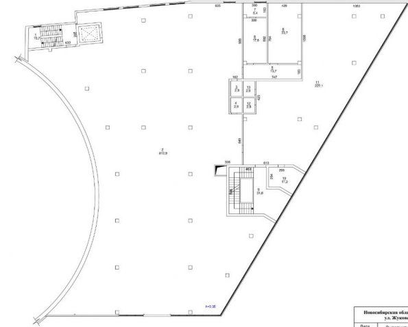
План части 2-го этажа
