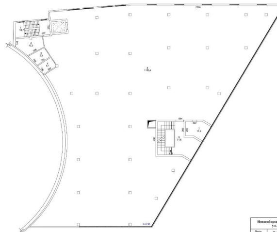
План части 3-го этажа
